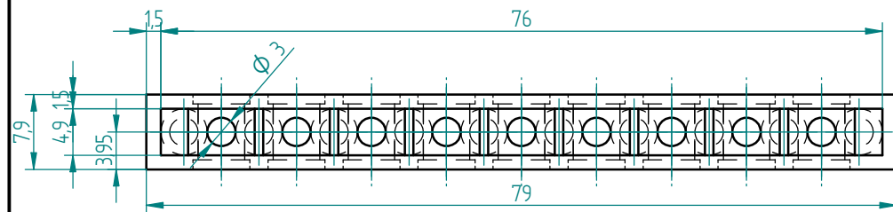
Lochleiste
